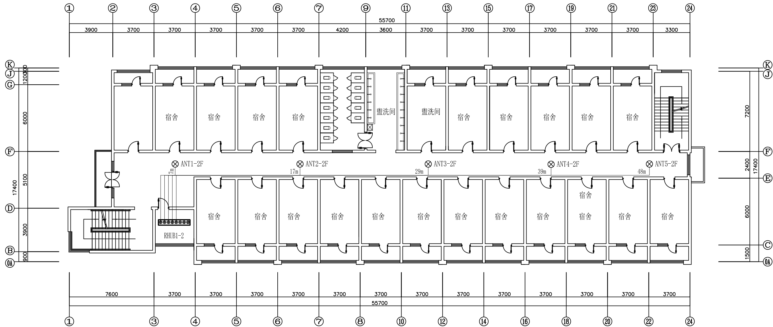
二-六层平面图
